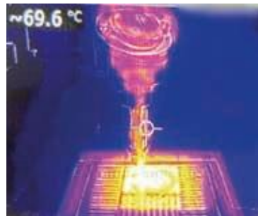
Riscaldamento di una sonda inserita in un calibratore a secco di tipo convenzionale.
