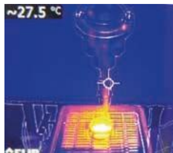
Riscaldamento di una sonda inserita in un Pyros 650 con dispositivo di ventilazione tangenziale
